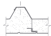
Detalle unión
